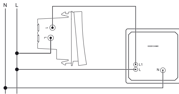
> Door Chime MLDRCHM2M_WH, MLDRCHM2M_AN
